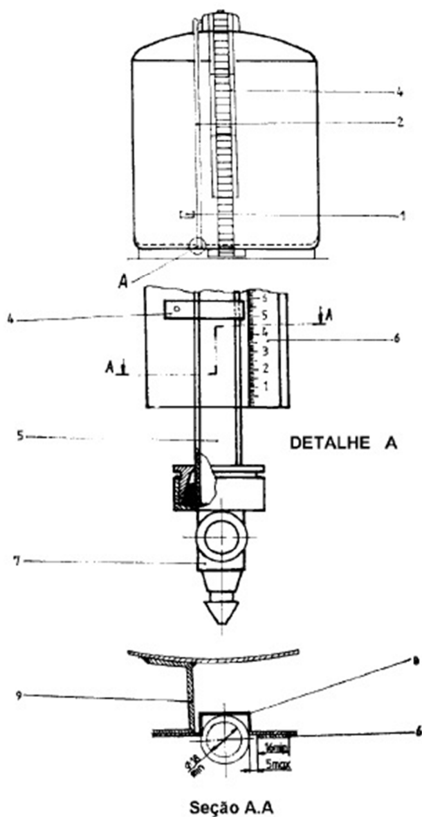
Figura 6 – Desenho esquemático de um tubo de nível num tanque cilíndrico vertical para vinho (tonel de vinho).
