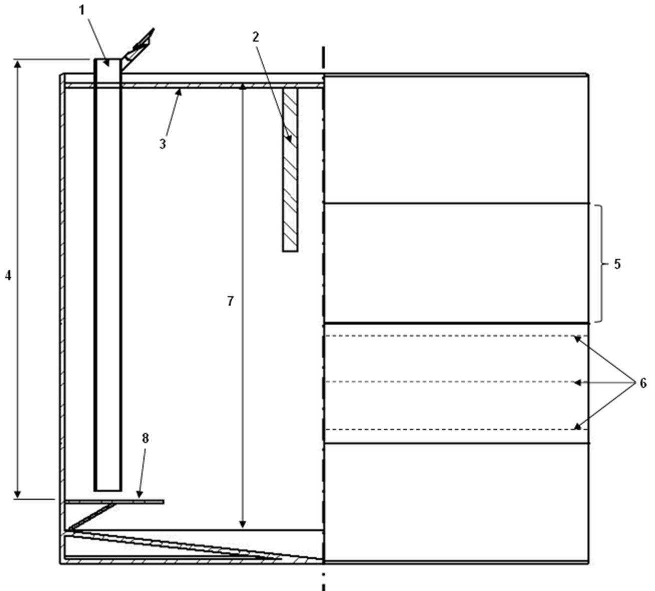
Figura 1 – Desenho esquemático de tanque cilíndrico vertical.
