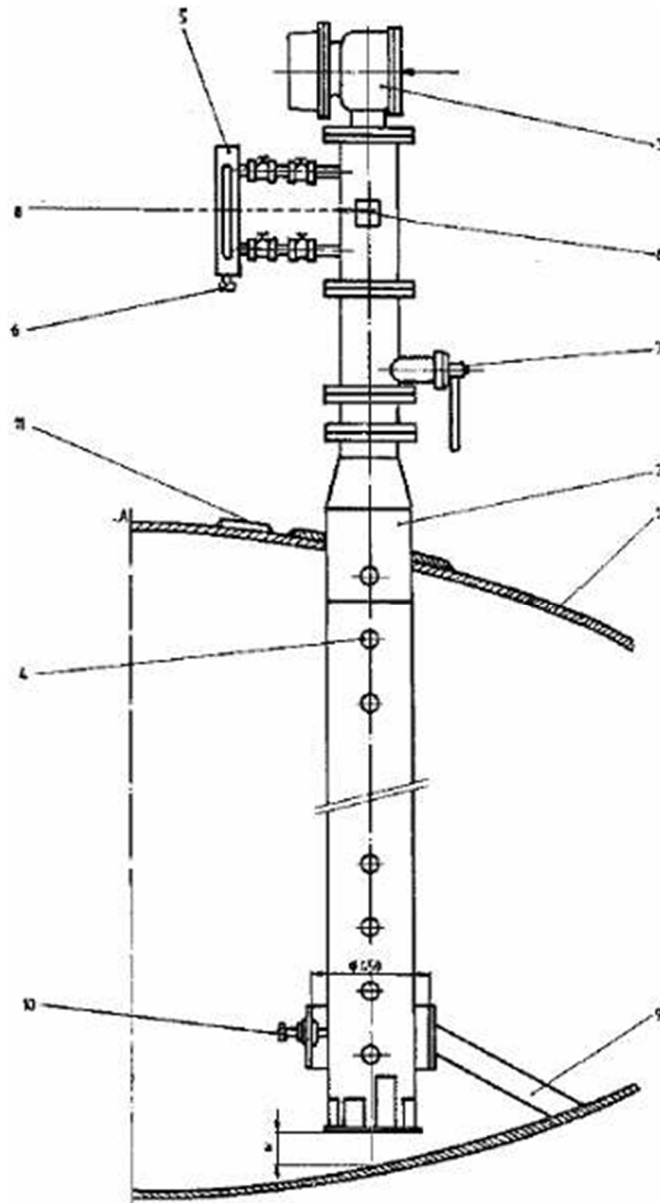
Figura 9 – Desenho esquemático de um tanque esférico pressurizado.
